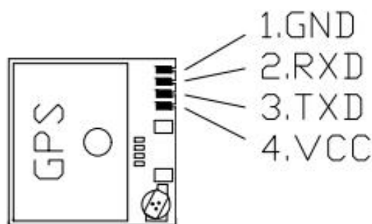
图 1：引脚分配
