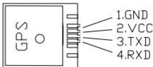
图 2：引脚分配
