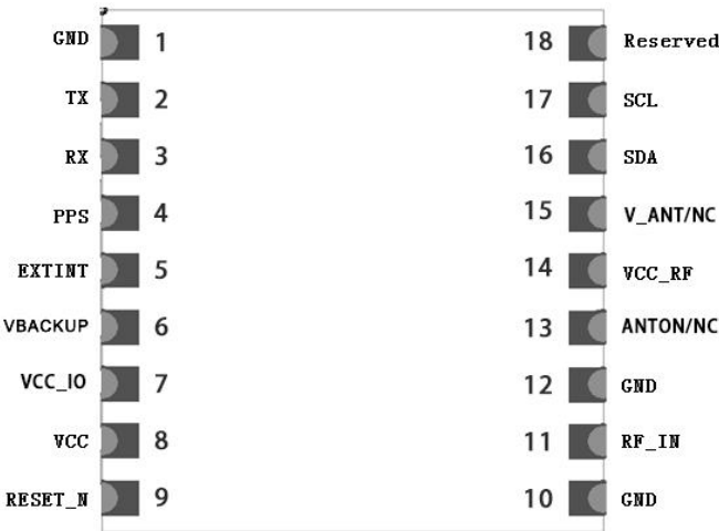
图 2: 引脚分布
