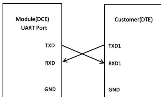
图 3:串口连接
